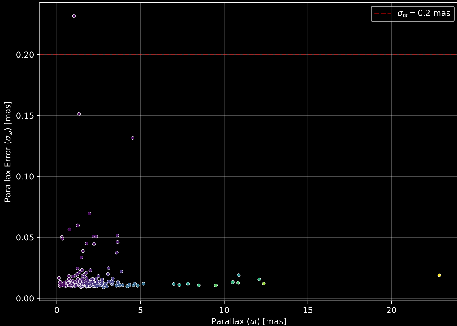
GALAH DR4 Field: [6886] Parallax Quality (n= 272)
