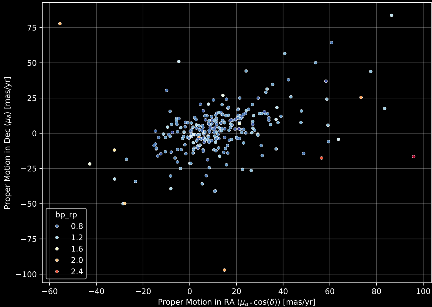
GALAH DR4 Field: [6886] Proper Motion Diagram (n= 272)
