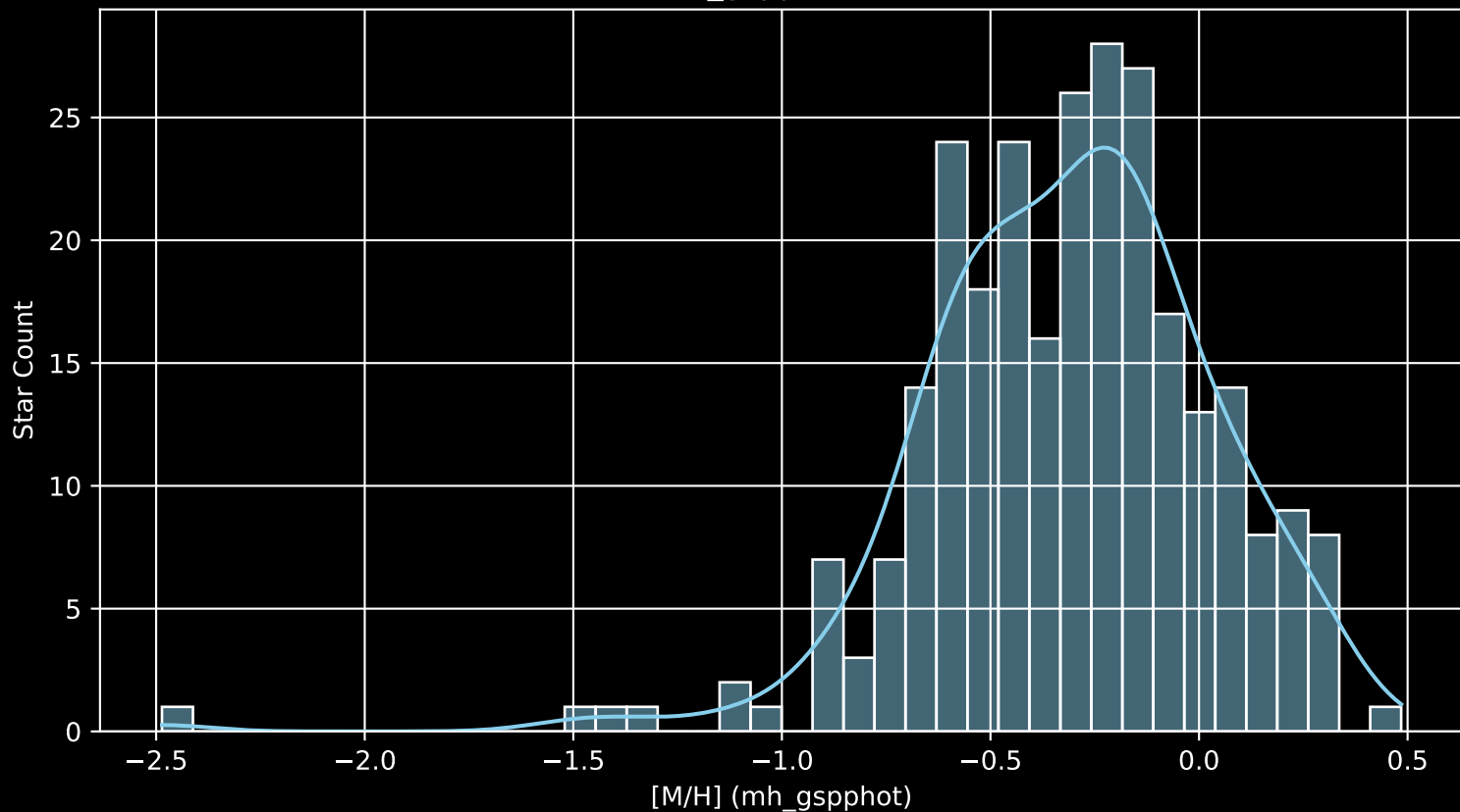
GALAH DR4 Field: [6886] [M/H] (mh_gspphot) (n= 271)
